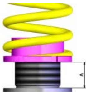
Restgewindemaß A bei Höhenverstellungen
