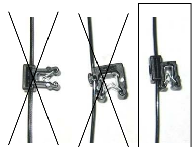
Edge Clips
