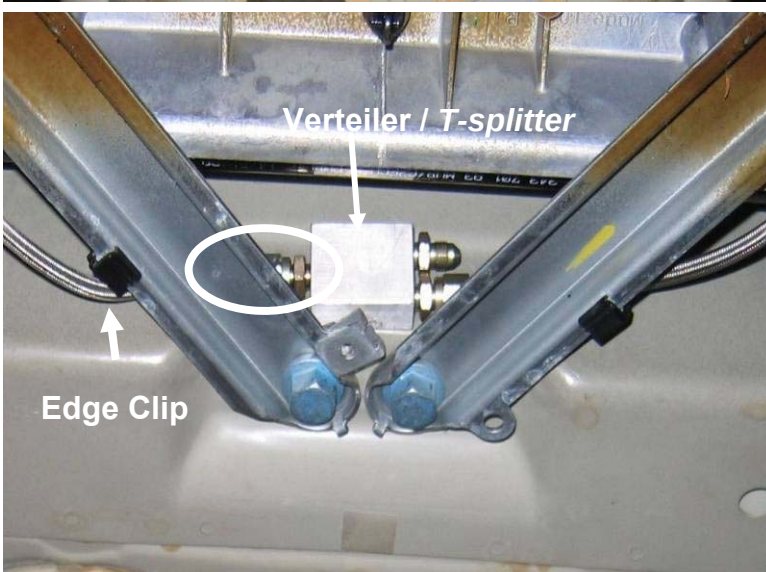
Edge Clips
