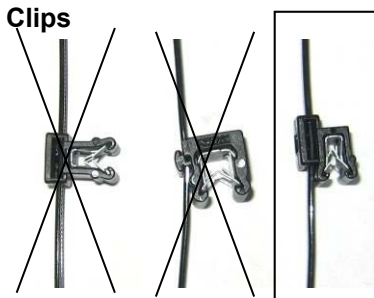
Edge Clips
