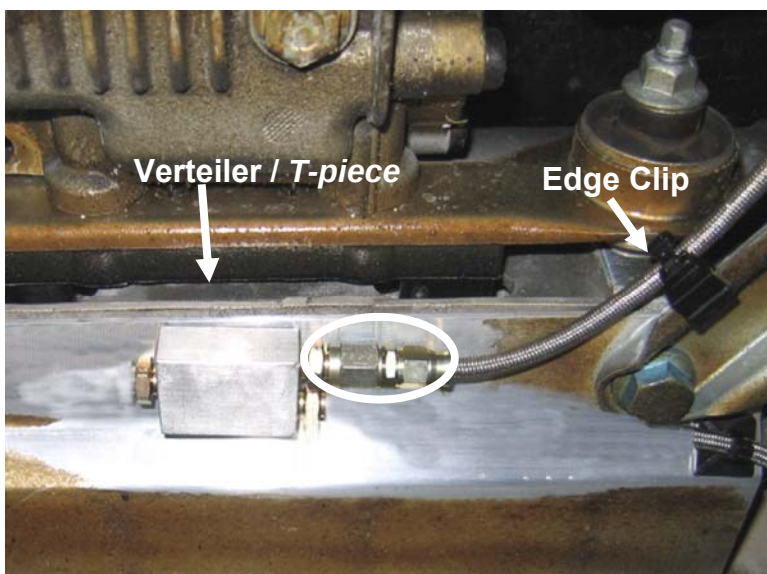
Edge Clips
