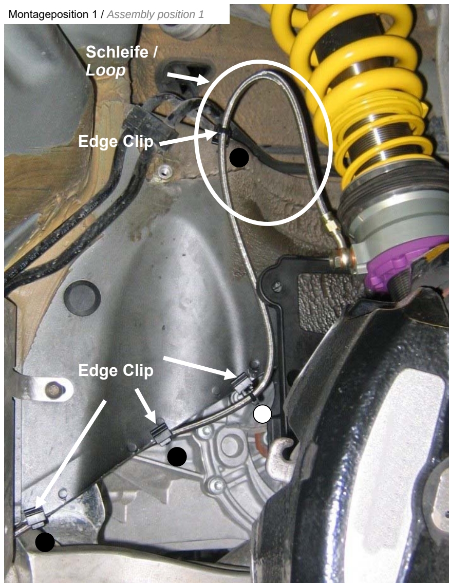
Edge Clip
